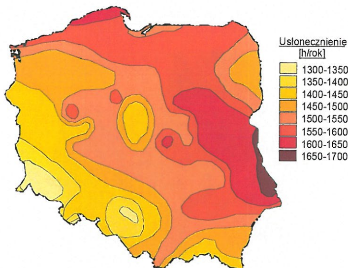
Rysunek 4 Średnie roczne sumy usłonecznienia
